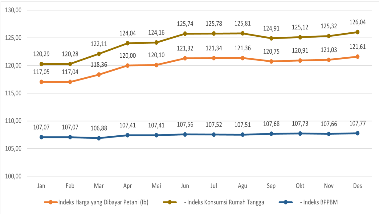
Gambar 4.4.5 Perkembangan Ib Kabupaten Tanah Bumbu dan Komponen Penyusunnya (IKRT dan Indeks BPPBM) Pada Tahun 2024
