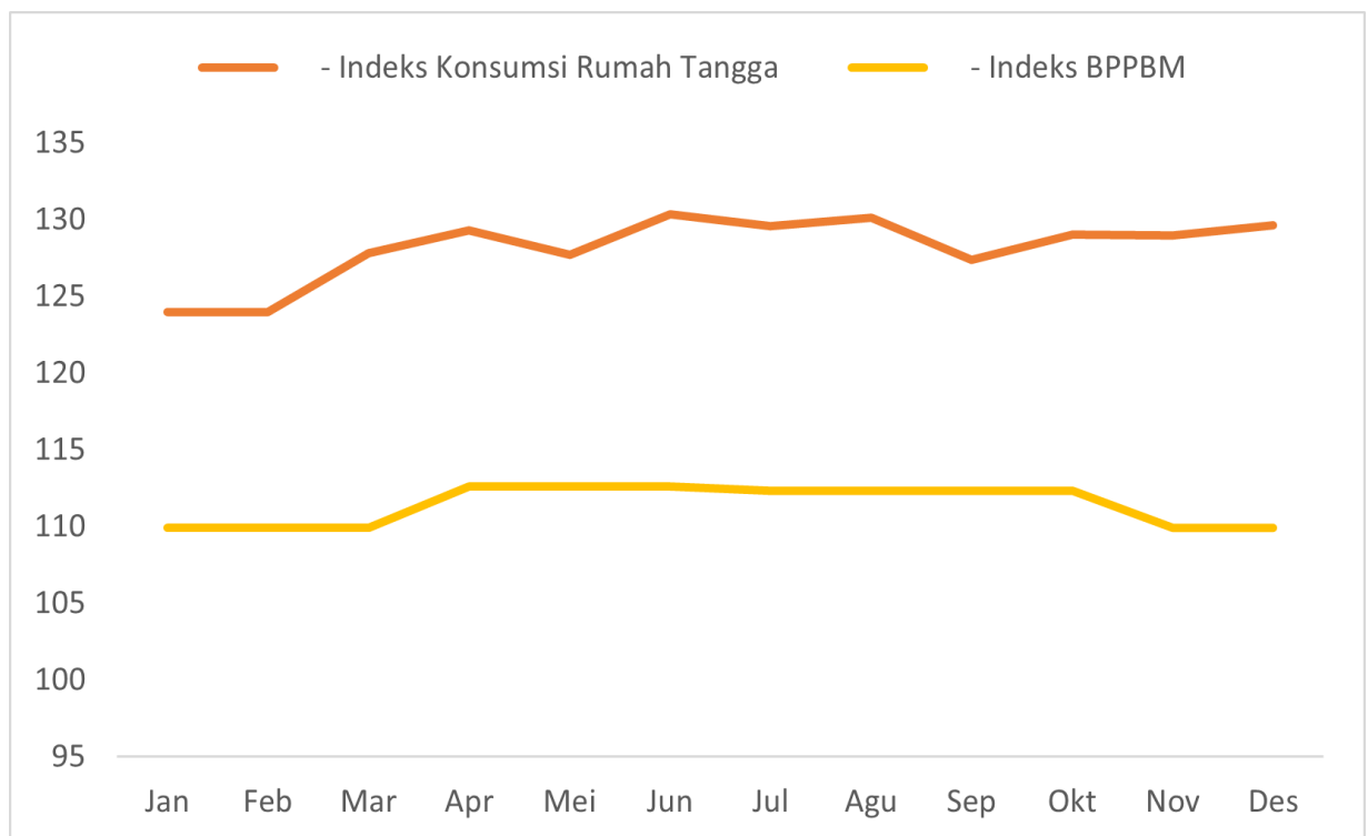
Gambar 4.3.2 Indeks Konsumsi Rumah Tangga dan Indeks Biaya Produksi dan Penambahan Barang Modal (BPPBM) Kabupaten Tanah Bumbu Tahun 2024
