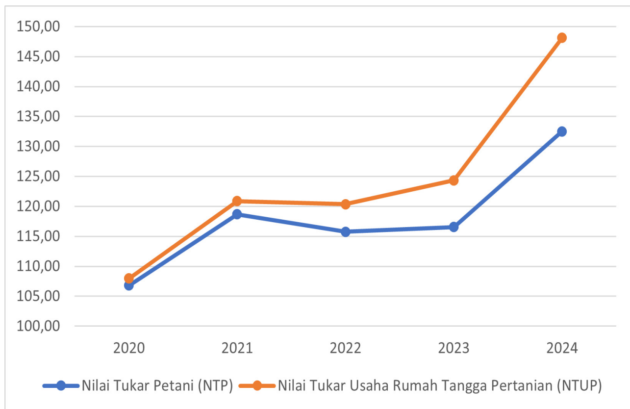
Gambar 4.6.5 Perkembangan NTP dan NTUP Kab. Tanah Bumbu Tahun 2020–2024
