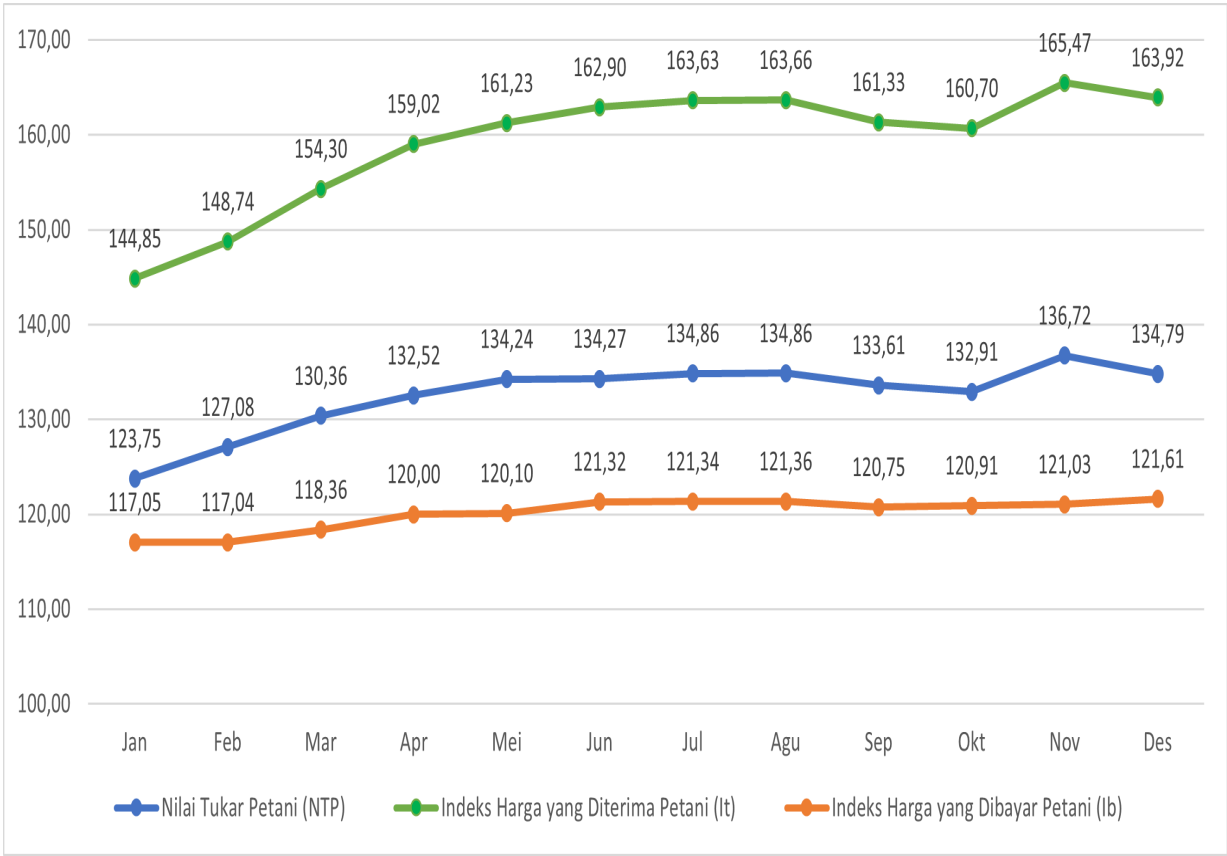
Gambar 4.4.3 Perkembangan Indeks Harga yang Diterima Petani (It), Indeks Harga yang Dibayar Petani (Ib), dan NTP Kabupaten Tanah Bumbu Pada Tahun 2024
