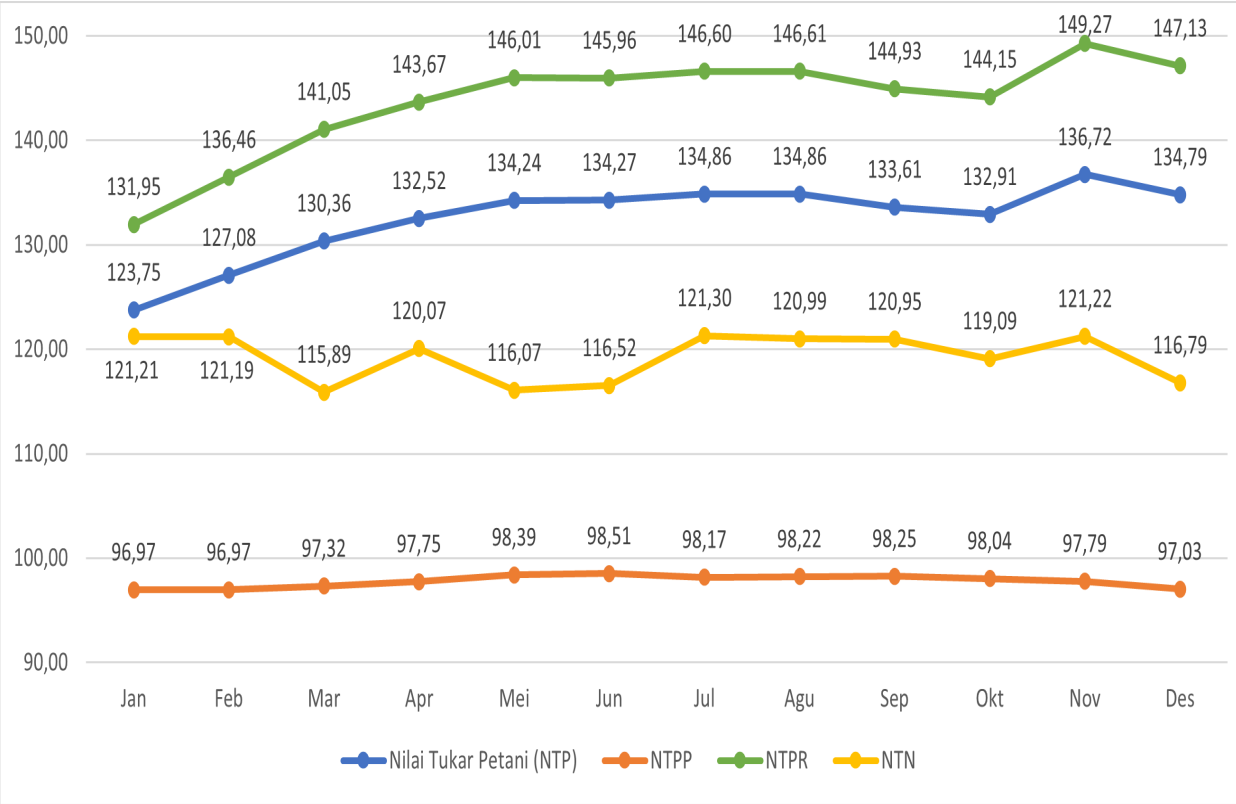
Gambar 4.4.2 Perkembangan NTP Kabupaten Tanah Bumbu, NTP Tanaman Pangan, NTP Perkebunan Rakyat, dan NTP Perikanan pada Tahun 2024
