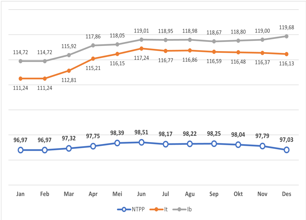
Gambar 4.1.1 NTPP, It dan Ib Kabupaten Tanah Bumbu Tahun 2024
