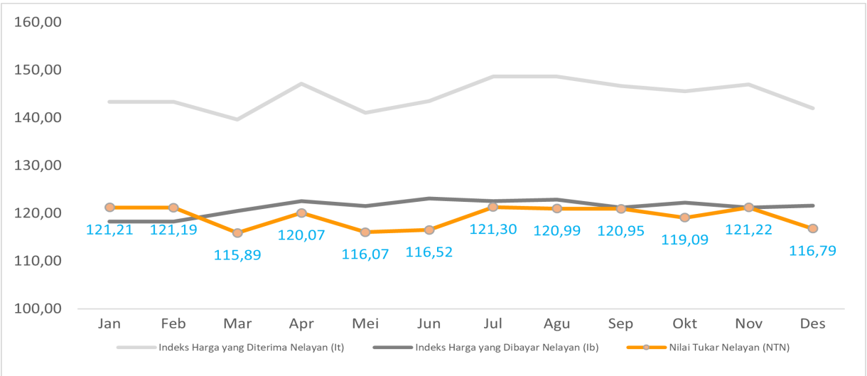
Gambar 4.3.1 It, Ib, dan NTN Kabupaten Tanah Bumbu Tahun 2024
