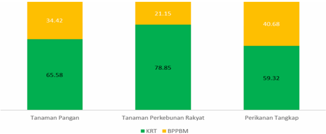
Gambar 4.4.1 Persentase Pengeluaran Konsumsi Rumah Tangga dan BPPBM menurut subsektor, Kabupaten Tanah Bumbu (2018=100)
