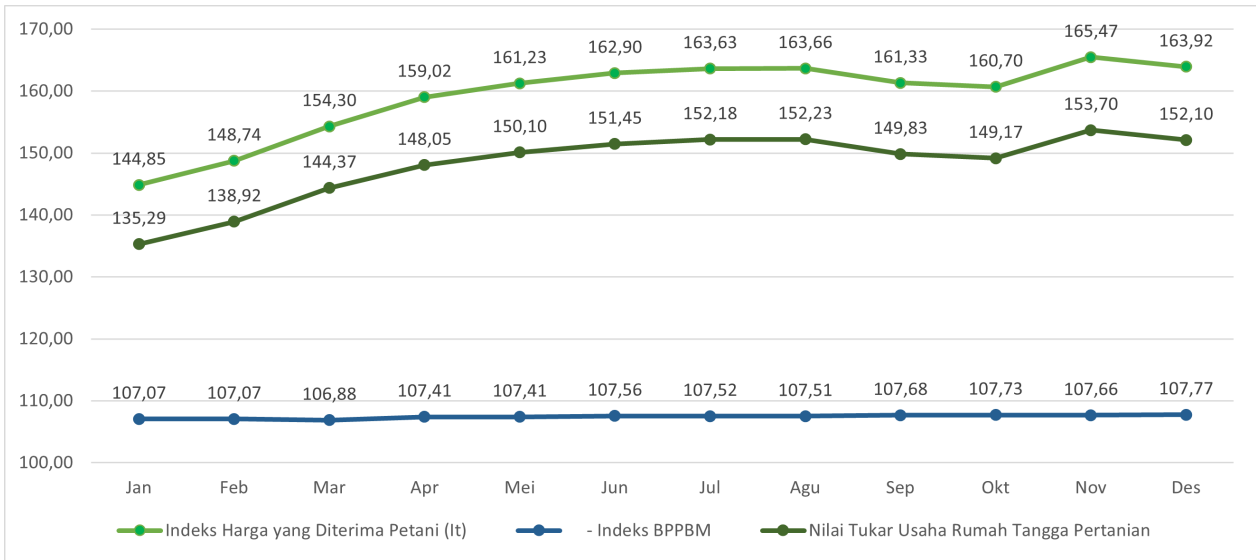
Gambar 4.5.1 Perkembangan NTUP, It dan Indeks BPPBM Kabupaten Tanah Bumbu Tahun 2024
