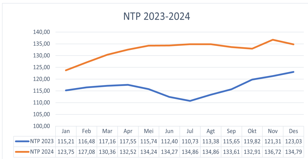
Gambar 4.6.1 Perkembangan NTP Kabupaten Tanah Bumbu setiap bulan pada Tahun 2023-2024 (a), Penyusun NTP Kabupaten Tanah Bumbu Tahun 2023 (b) dan Penyusun NTP Kabupaten Tanah Bumbu Tahun 2022 (c).
