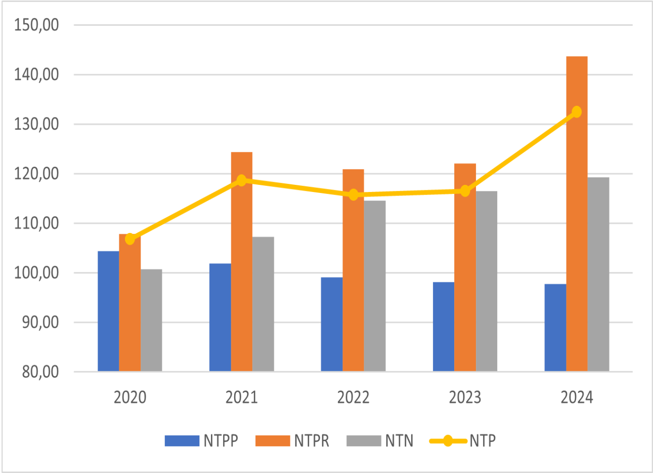
Gambar 4.6.4 Perkembangan NTP, NTPP, NTPR dan NTN Kab. Tanah Bumbu Tahun 2020–2024
