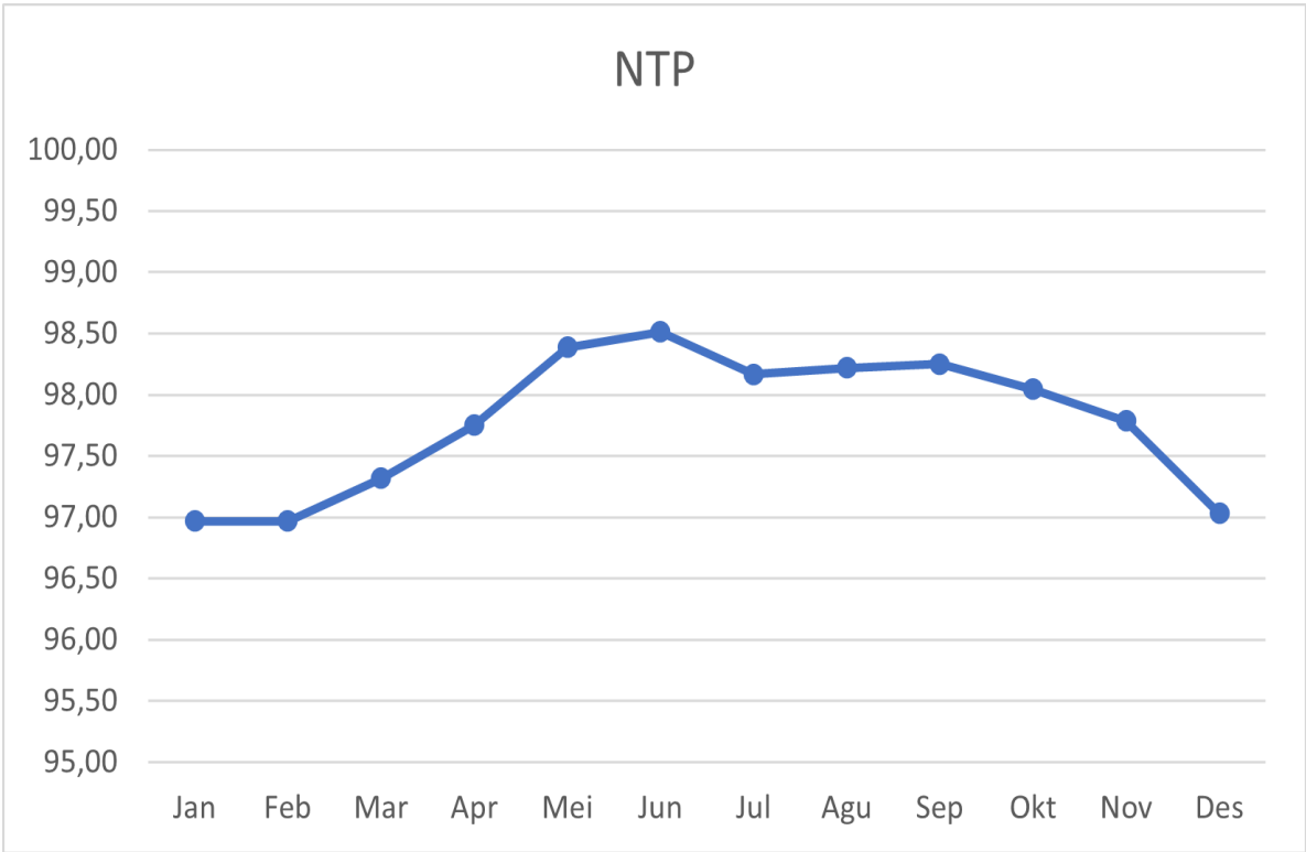
Gambar 4.1.2 NTPP Kabupaten Tanah Bumbu Tahun 2024
