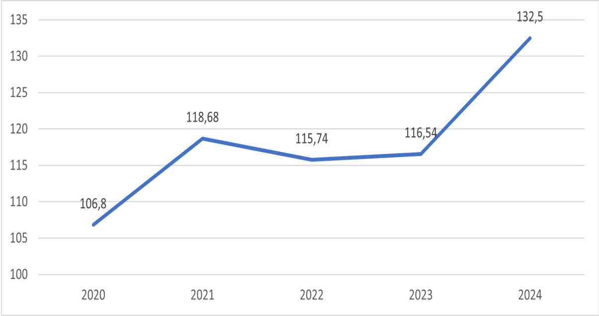
Gambar 4.6.2 Rata-rata NTP Kabupaten Tanah Bumbu, Tahun 2020-2024
