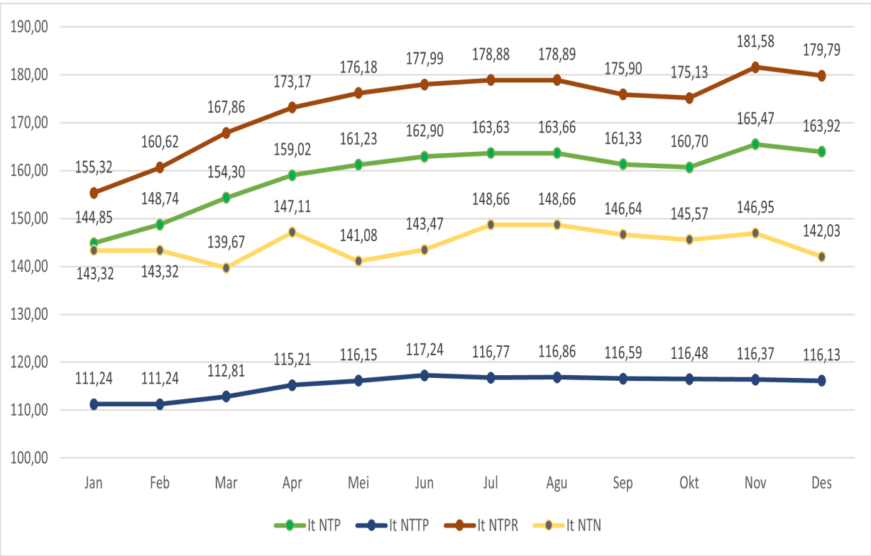
Gambar 4.4.4 Perkembangan It Kabupaten Tanah Bumbu, It Tanaman Pangan, It Perkebunan Rakyat, dan It Perikanan Tangkap Pada Tahun 2024
