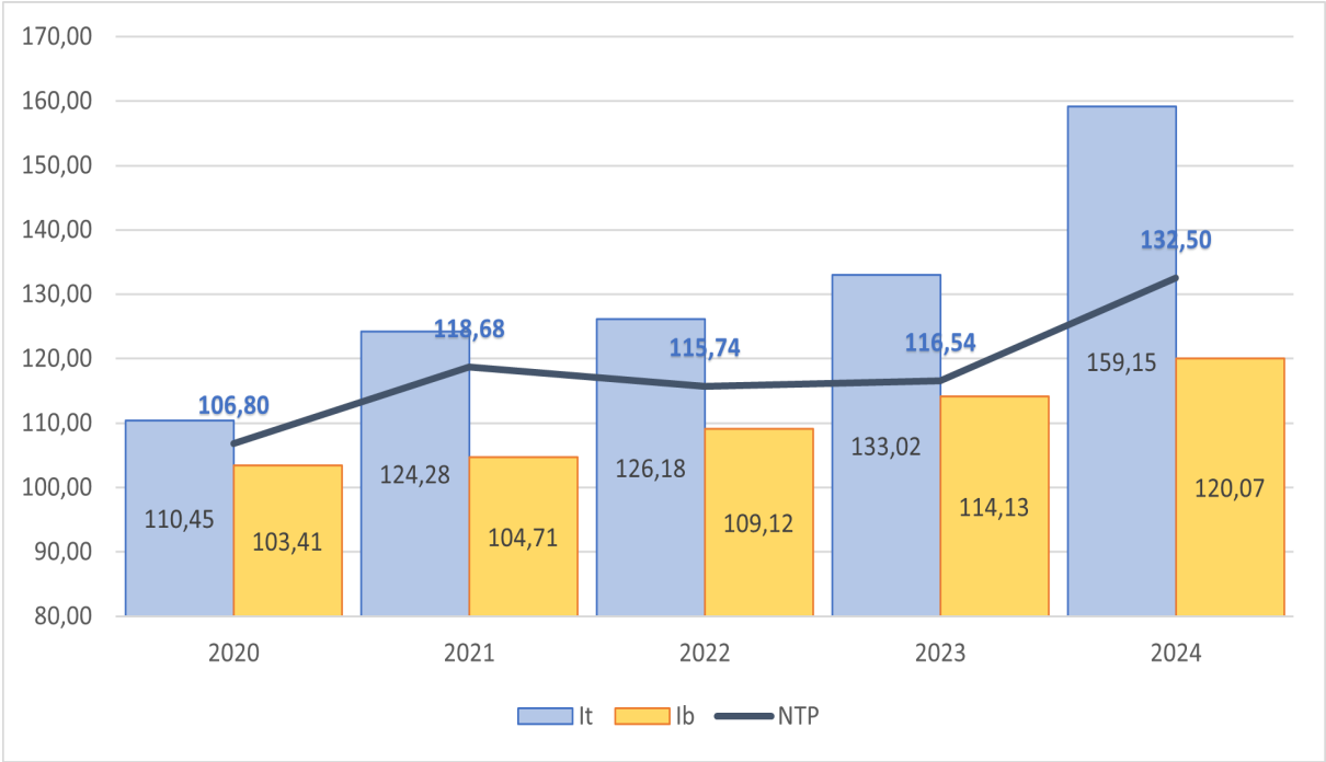
Gambar 4.6.3 Perkembangan It, Ib dan NTP Kab. Tanah Bumbu Tahun 2020–2024
