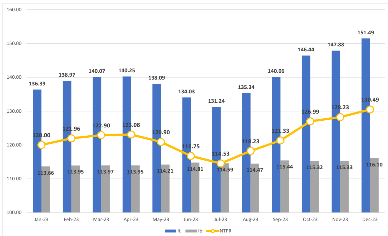
Gambar 4.2.1 It, Ib, dan NTPR Kabupaten Tanah Bumbu Tahun 2024
